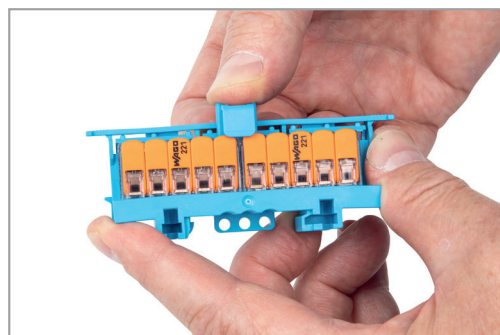
Einsetzen des Brückers mit Verriegelungsfunktion in geschlossene Klemmstellen
