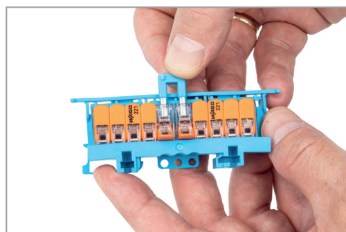
Entfernen des Brückers aus geöffneten Klemmstellen
