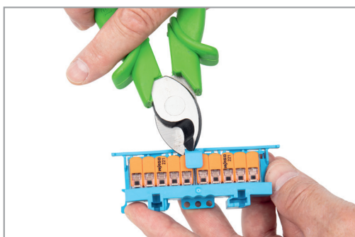
Nur notwendig bei Brücker mit Verriegelungsfunktion Entfernen der Verriegelung zum Zweck der bewussten Entnahme des Brückers
